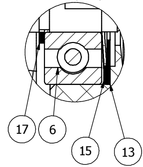
PARTICOLARE C (2:1)
